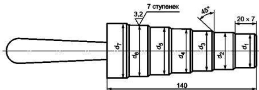
Рисунок 1 - Ступенчатый калибр
